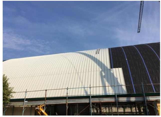
Posa del tetto in lamiera grecata (terzo strato del pacchetto di copertura)
